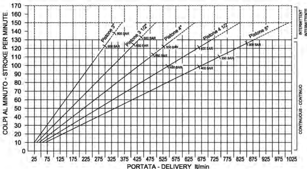
DIAGRAMMA PRESTAZIONI - PERFORMANCE DIAGRAM
